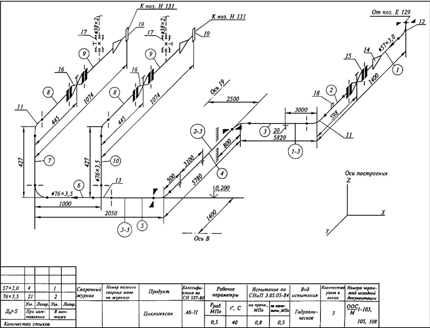
Деталировочный чертеж технологического трубопровода, выполняемого с разбивкой на элементы, специфицируемые по системе шифровки
