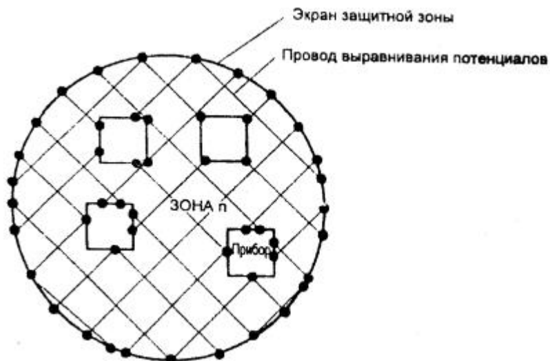
Рисунок 4.5 - Сетчатое выполнение системы выравнивания потенциалов
