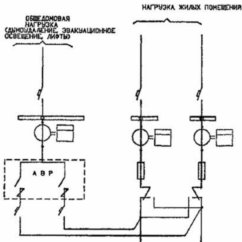
РИС. 2. СХЕМА УЧЕТА ЭЛЕКТРОЭНЕРГИИ В ЖИЛЫХ ДОМАХ 10 ЭТАЖЕЙ И ВЫШЕ
