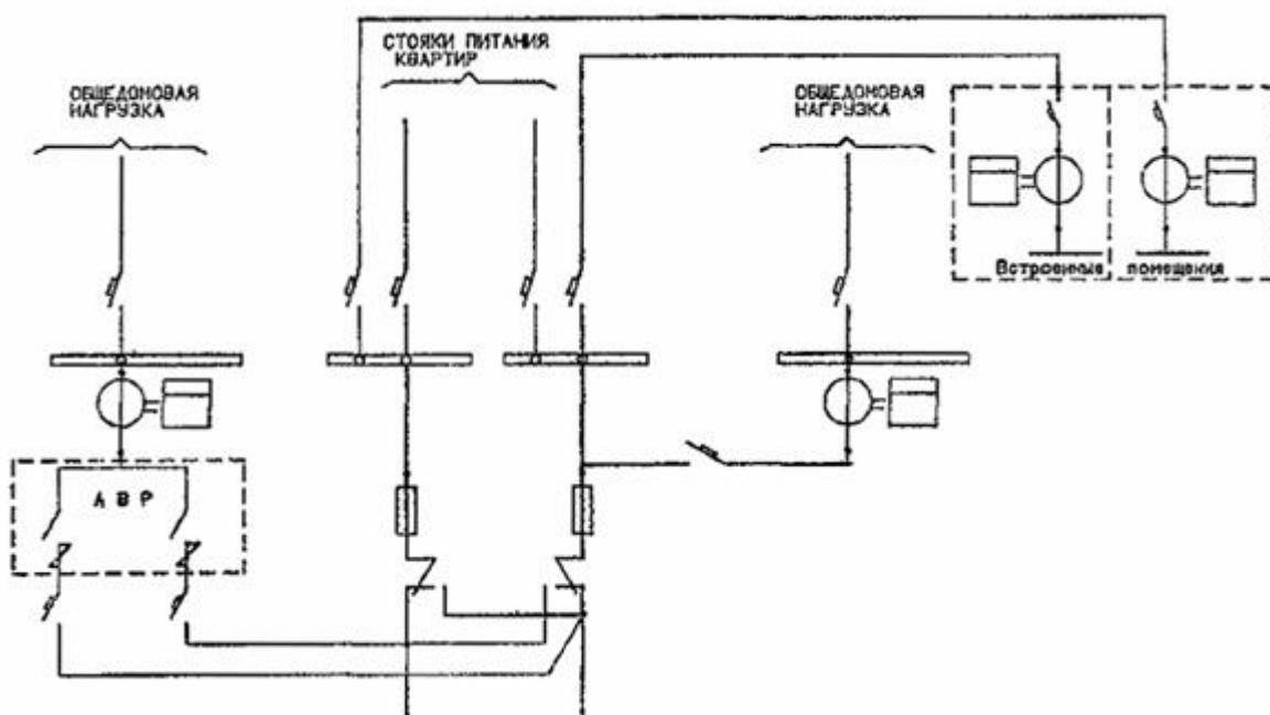
РИС. 2. СХЕМА УЧЕТА ЭЛЕКТРОЭНЕРГИИ В ЖИЛЫХ ДОМАХ 10 ЭТАЖЕЙ И ВЫШЕ
