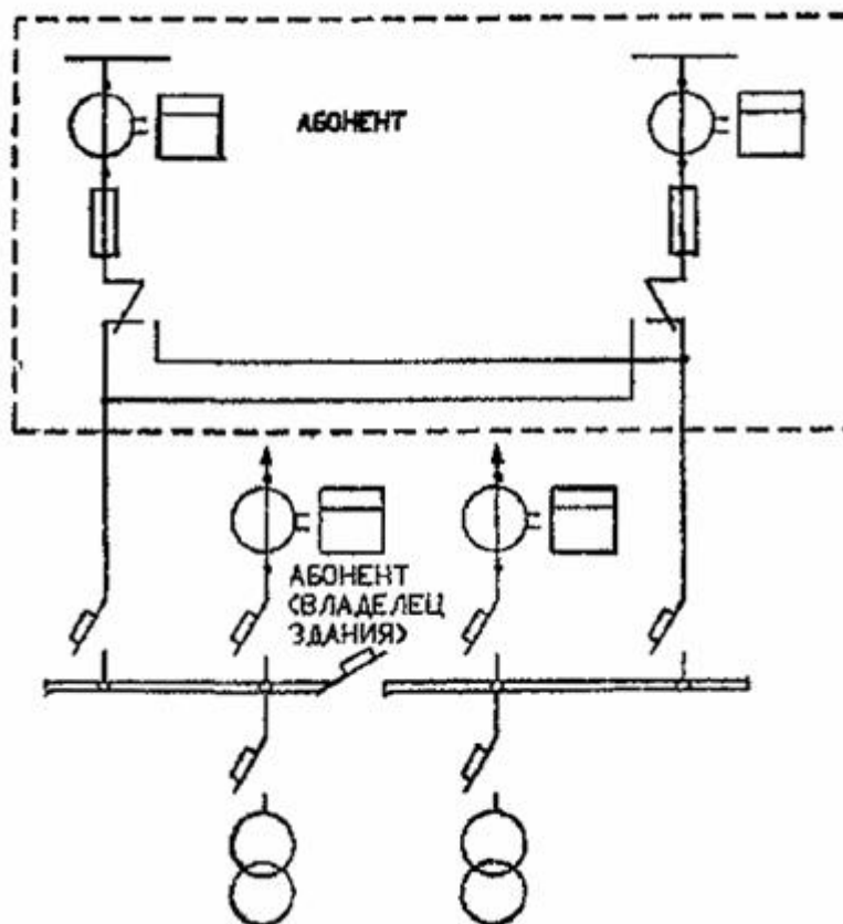
РИС. 4. СХЕМА УЧЕТА ЭЛЕКТРОЭНЕРГИИ В ОБЩЕСТВЕННЫХ ЗДАНИЯХ С НЕСКОЛЬКИМИ ПОТРЕБИТЕЛЯМИ
