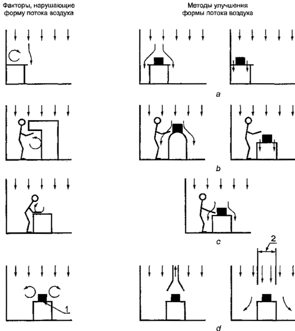
a - за счет лучшего расположения оборудования; b - за счет лучшей формы оборудования и рабочего места; c - за счет правильного поведения персонала; d - за счет специальной организации потоков воздуха; 1 - источник тепла; 2 - локальный поток с повышенной скоростью
